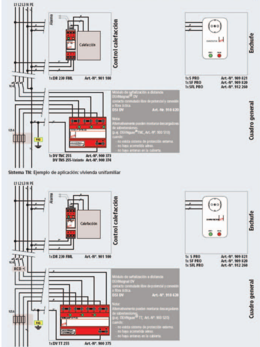
Sistema TT. Vivienda Unifamiliar.
