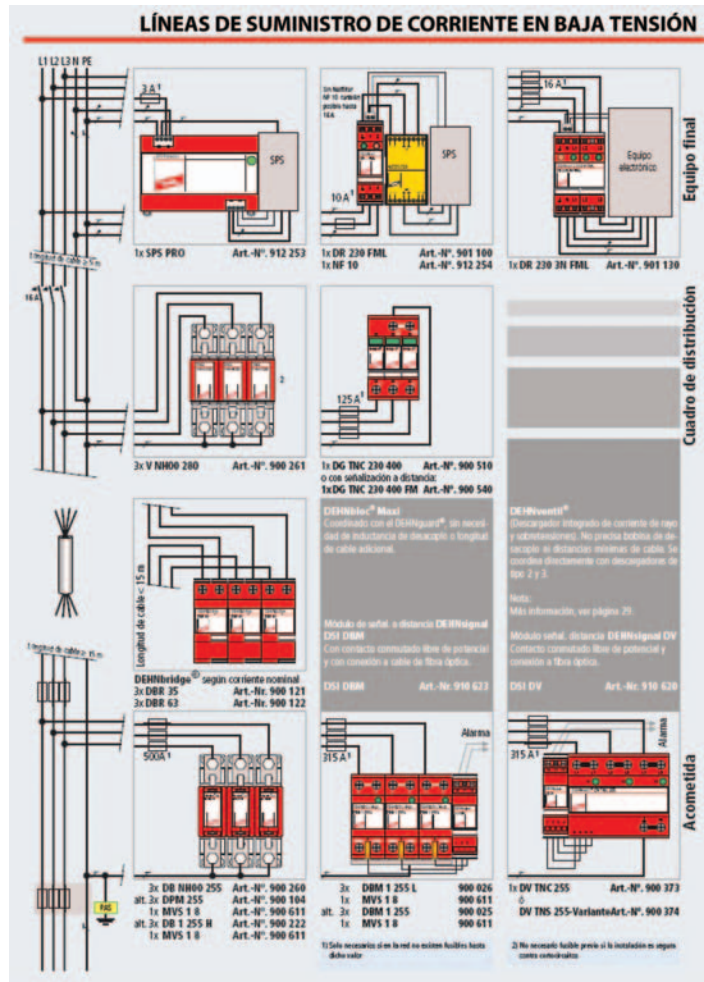
Sistema TN. Oficinas: Tendido separado de los conductores N y PE desde cuadro de distribución.
